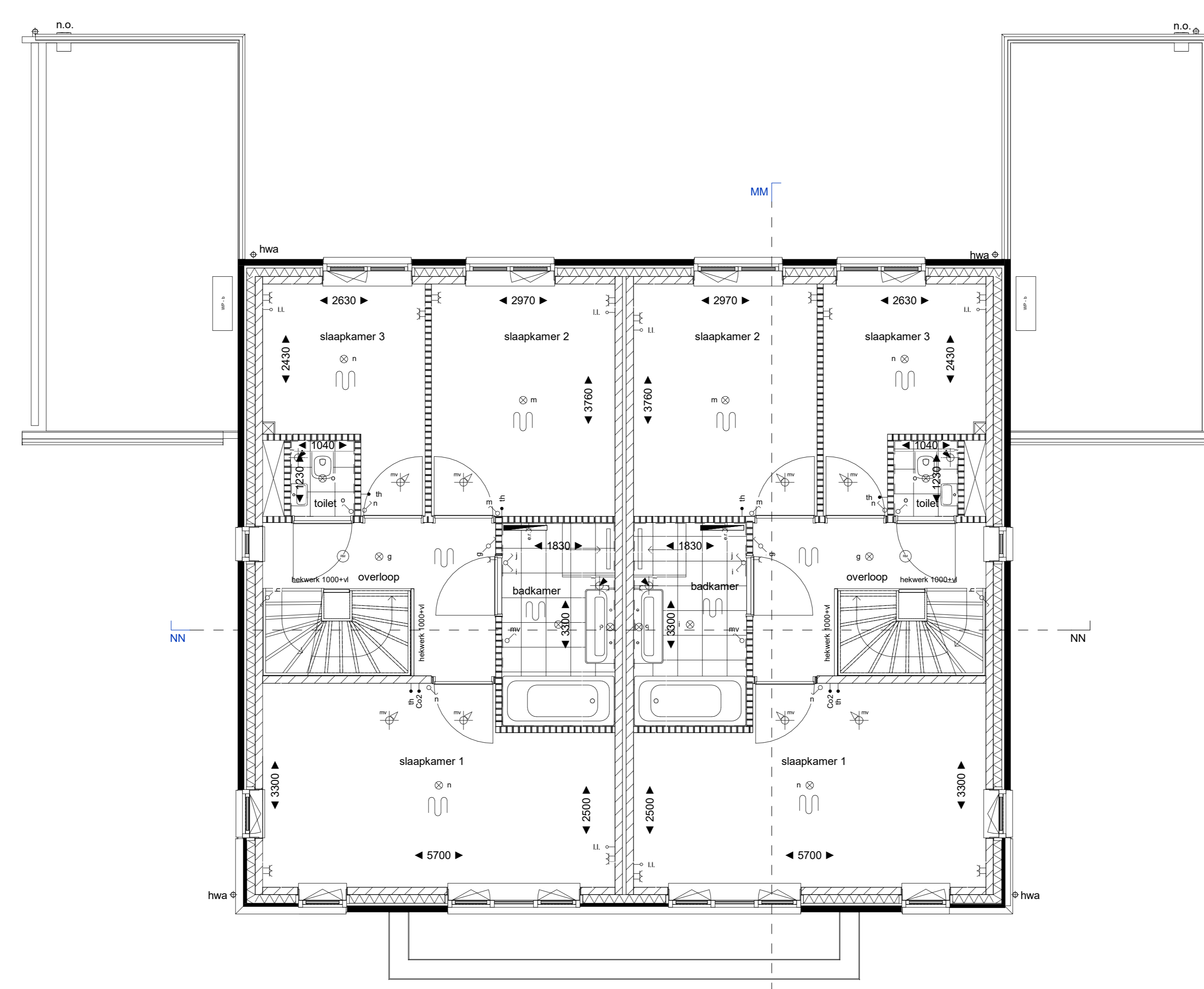
bwnr. 31 - Type D bwnr. 32 - Type Csp eerste verdieping
