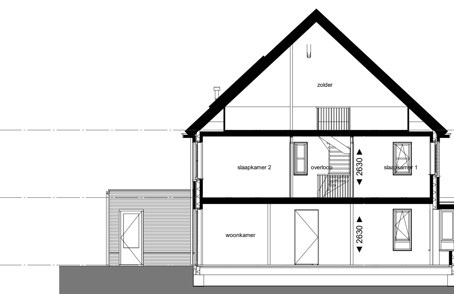
Doorsnede MM bwnr. 32 - Type Csp
