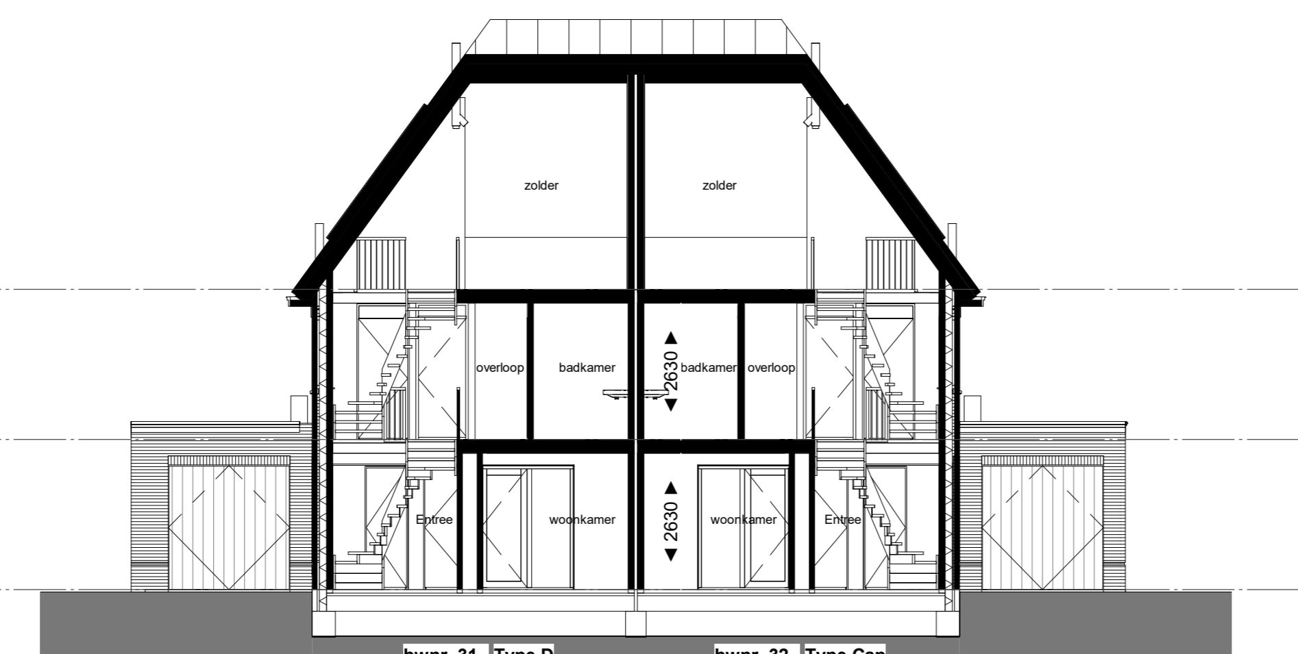
Doorsnede NN bwnr. 31 - Type D bwnr. 32 - Type Csp
