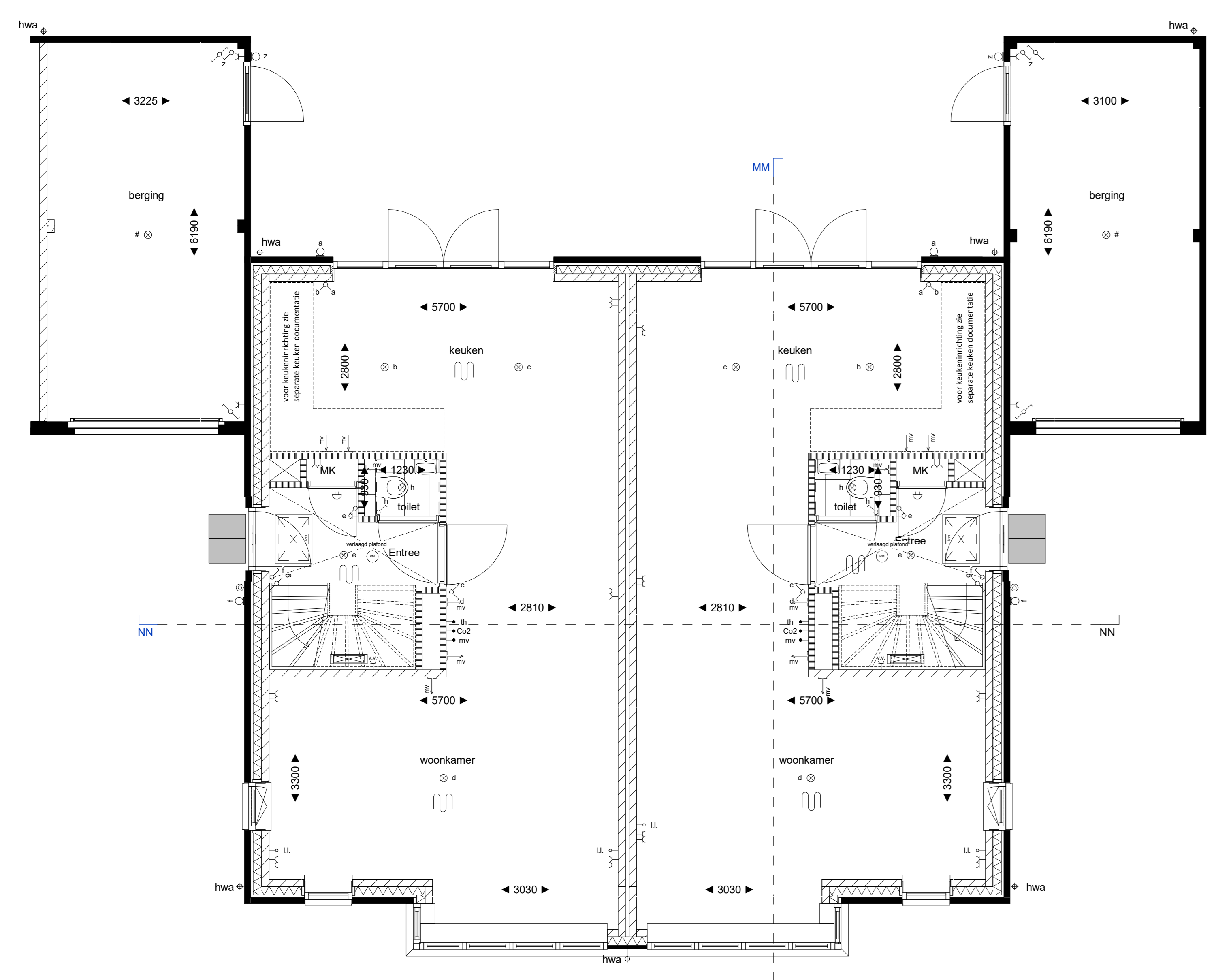
bwnr. 31 - Type D bwnr. 32 - Type Csp begane grond
